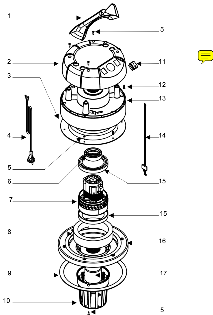
Complete motor head, Tête complète, Motorkopf kpl. Testa completa
