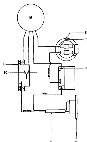
Verdrahtungs - Schema
